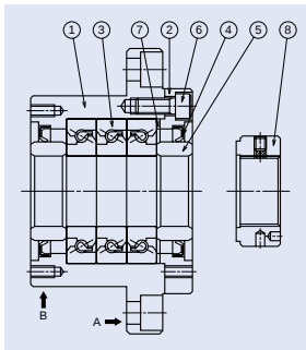
Детали опорного узла
