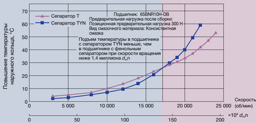
Результат эксплуатационных испытаний сепаратора
