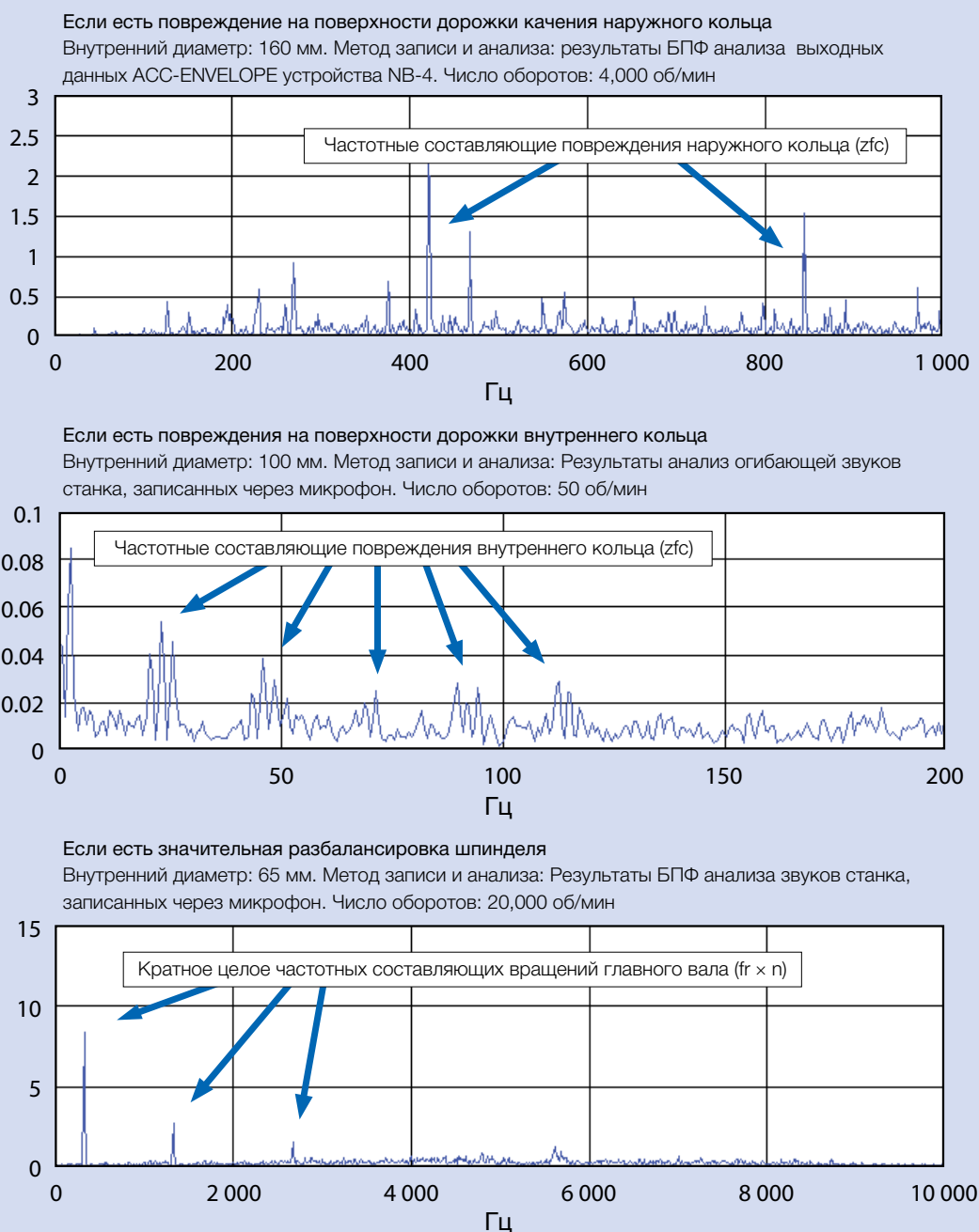
Рис. 2.4 Примеры результатов частотного анализа звуков и вибраций, проведенного при помощи программного обеспечения БПФ
