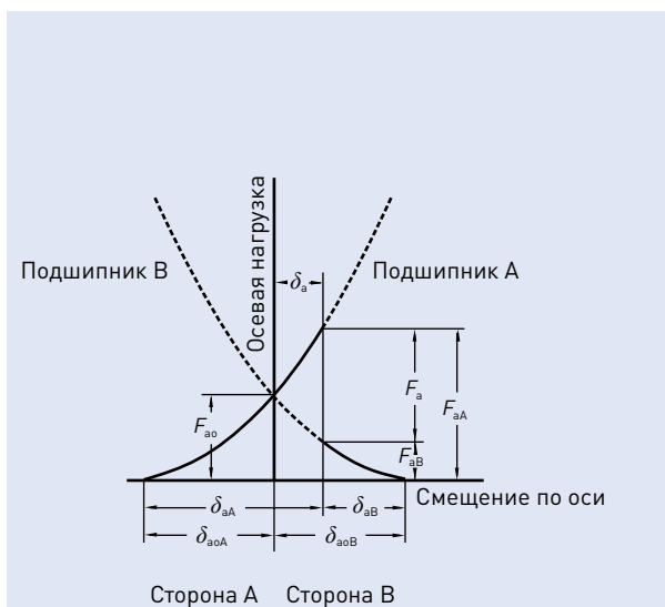
Рис. 4.4 Смещение по оси компоновки DB с преднатягом
