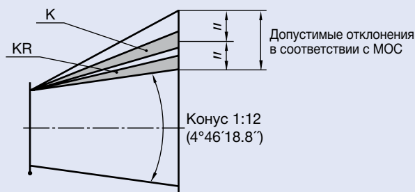
Рис. 7.2 Допустимые отклонения
