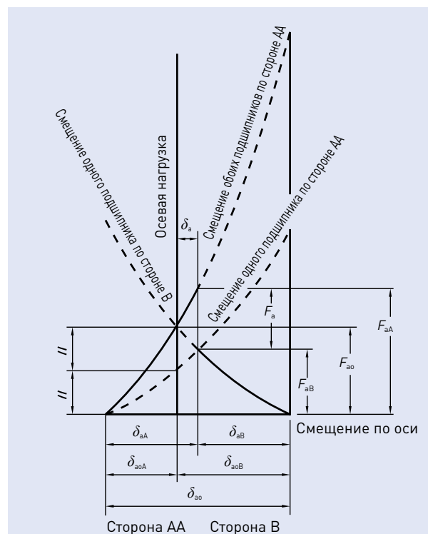
Рис. 4.6 Смещение по оси компоновки DBD с преднатягом
