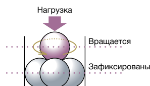
Испытание 4 шариков
