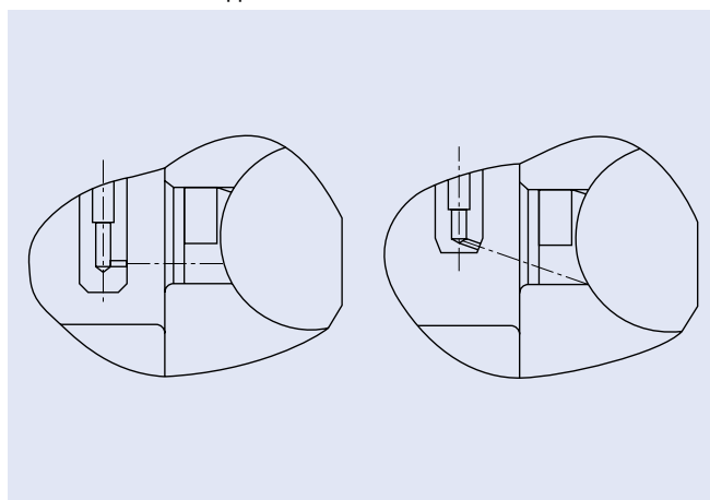
Рис. 9.1 Угол насадки
