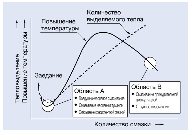
Рис. 6.1 Количество смазки и повышение температуры
