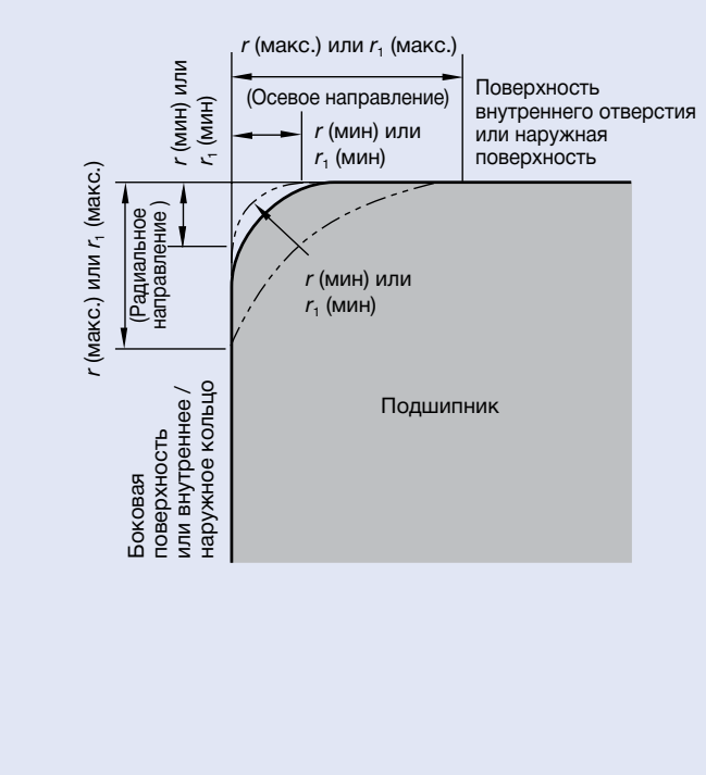
Рис. 8.2 Размеры фаски
