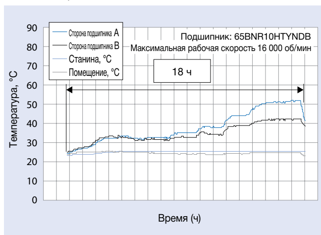
Рис. 3.1 Изменения температуры при работе с постоянной скоростью
